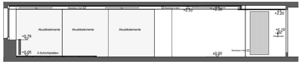
Schnitt B-B
