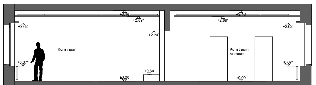
Schnitt B-B
